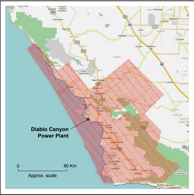
a. Aeromagnetic Survey Area 2008
